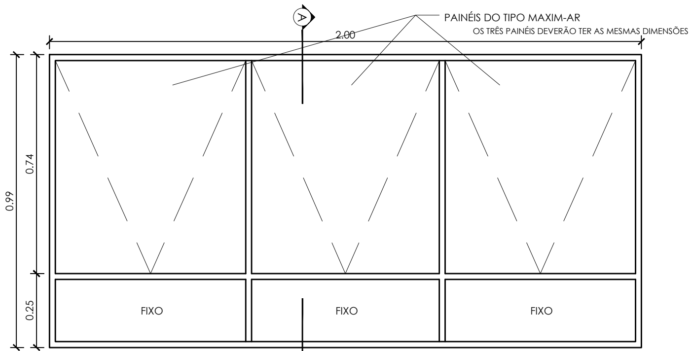
1 VISTA EXTERNA SEM ESCALA
